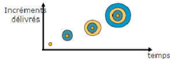
modèle incrémental
