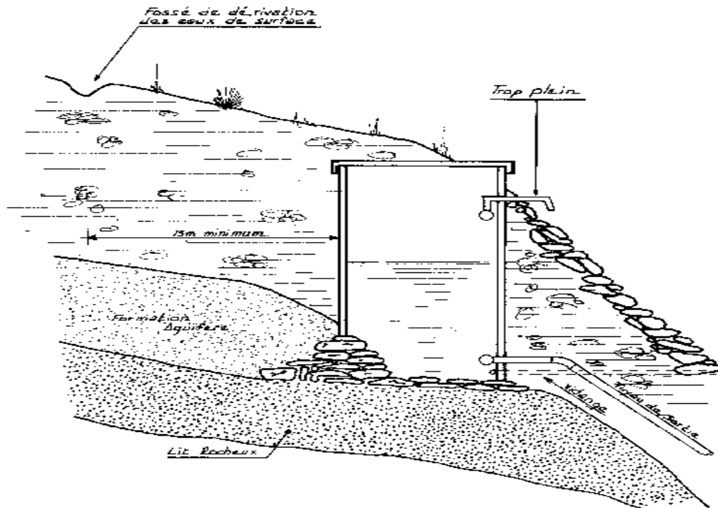
Figure 1.11. Schéma d'aménagement avec réservoir (Source : Comité Interafricain d'Etudes hydrauliques)
