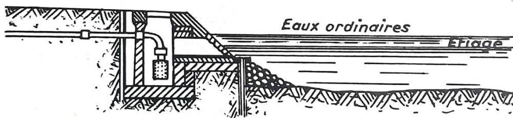
Figure 1.7. Prise en rivière par l'intermédiaire d'un puits
