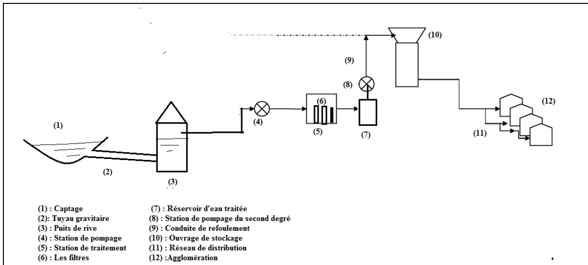
Figure 1.5. Schéma d'alimentation en eau potable : source superficielle
