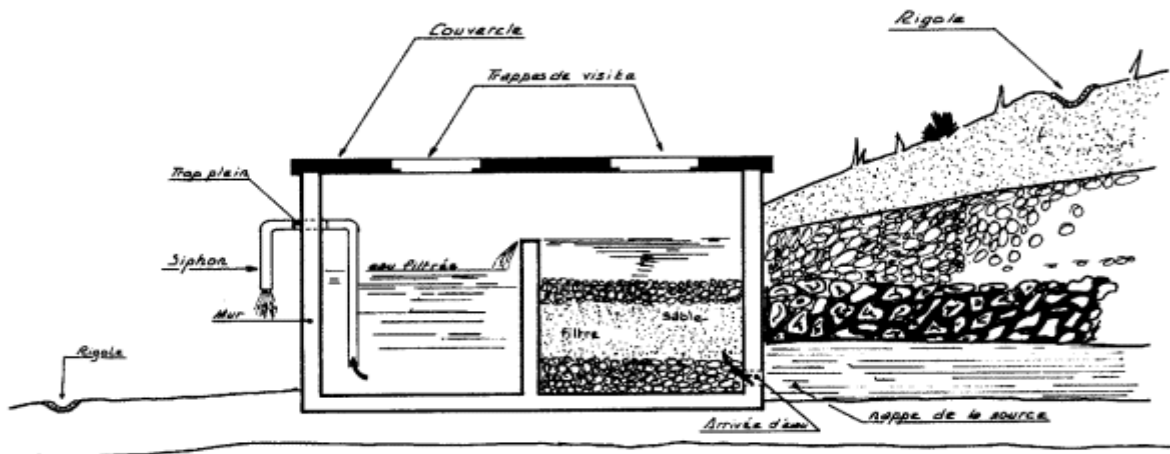
Figure 1.12. Schéma d'aménagement avec réservoir et filtre (Source : Comité Interafricain d'Etudes hydrauliques)
