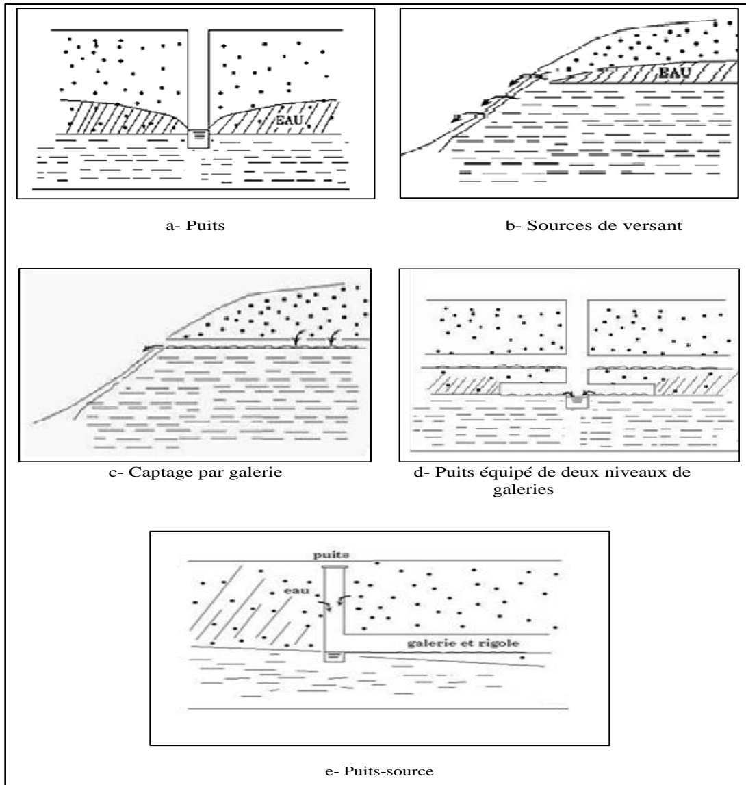
Figure 1.14. Différents types de captage des eaux souterraines
