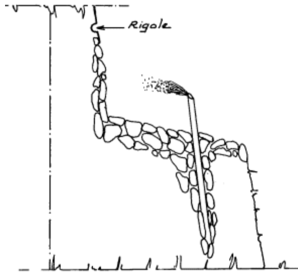
Figure 1. 10. Schéma d'aménagement simple d'une source (Source : Comité Interafricain d'Etudes hydrauliques)
