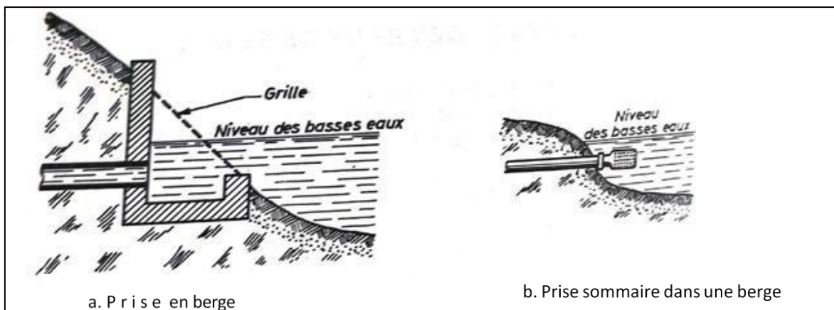
Figure 1. 8. Prise en berge
