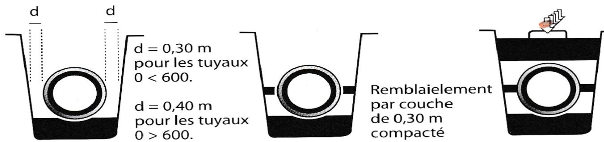
Figure 1.3. Pose et remblais des conduites en béton( Guide technique -Alcahyd)
