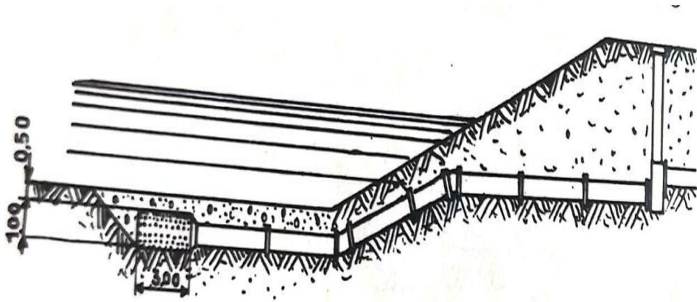
Figure 1.9. Prise d'eau sous le lit d'une rivière
