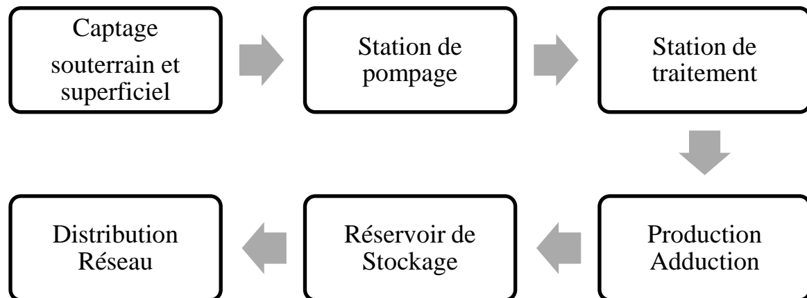
Figure 1.1. Schéma général d'un réseau d'A.E.P
