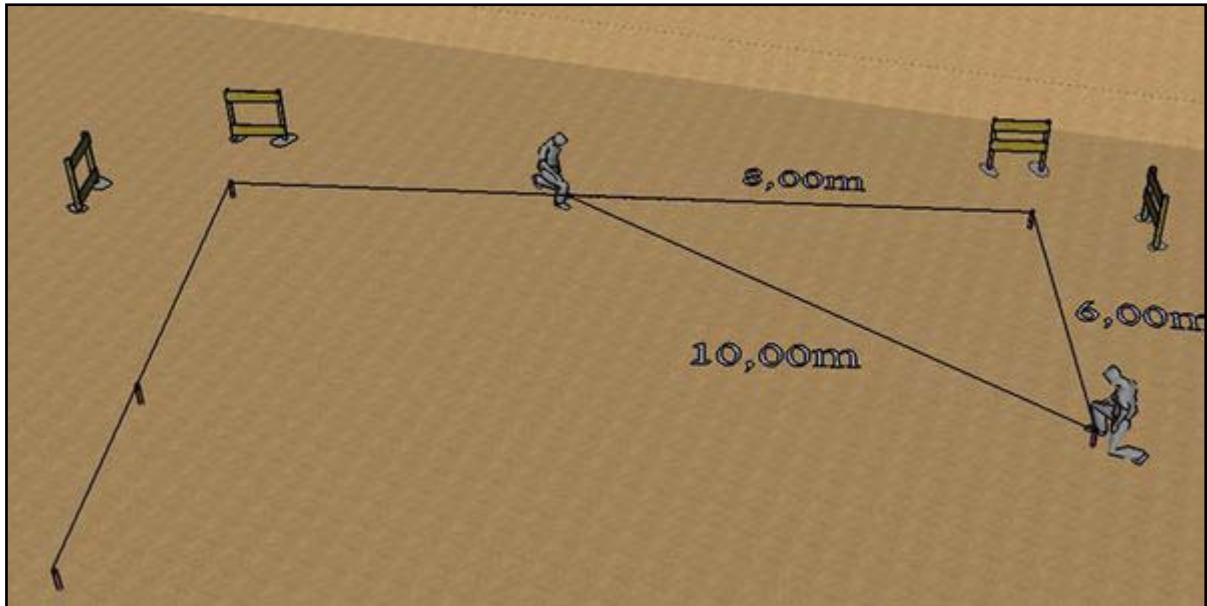
Figure 5 : Procédé de réalisation d'une équerre sur chantier
