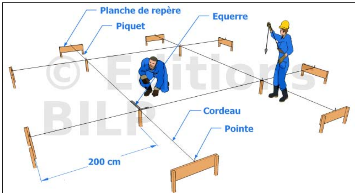
Figure 6 : Exemple de mise en place de chaises d'implantation
