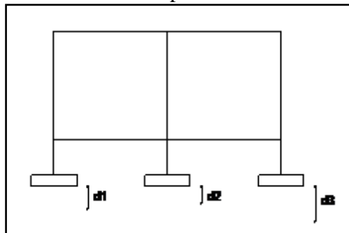
Figure 02 : illustration d'un tassement différentiel
