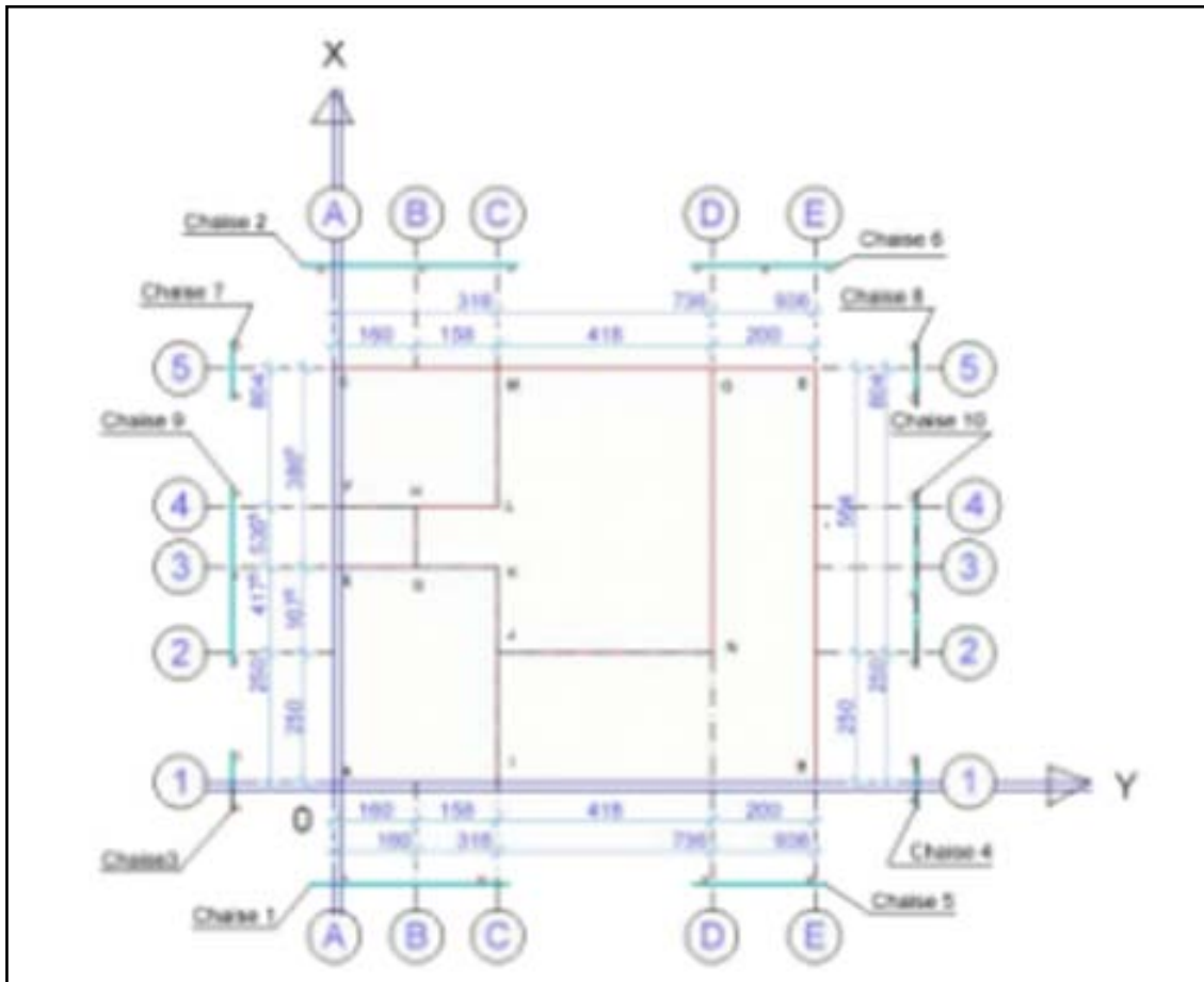
Figure 4 : Contenu d'un plan d'implantation
