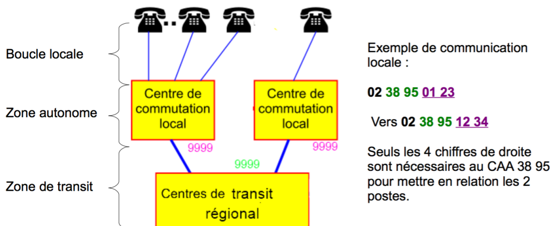
Figure II.9. Exemple d'une communication locale
