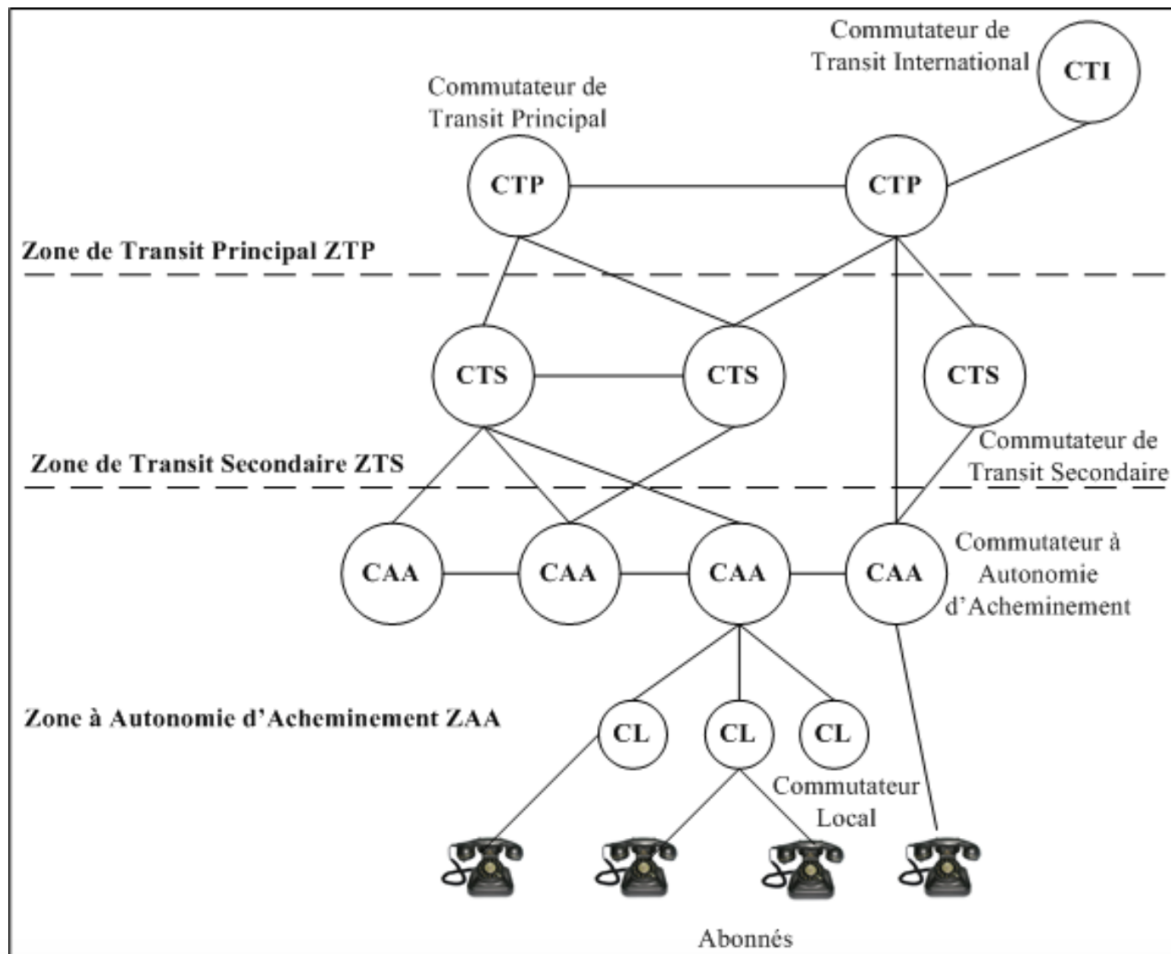
Figure II.8. Schéma simplifié d'un tronçon du réseau RTC
