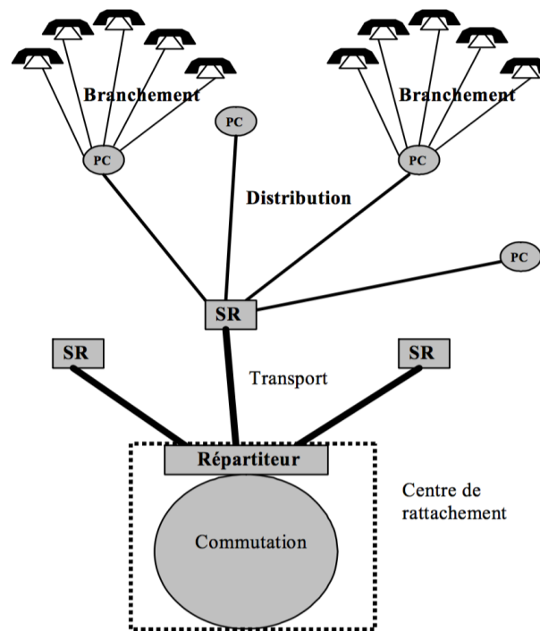
Figure II.3. Structure de réseau local
