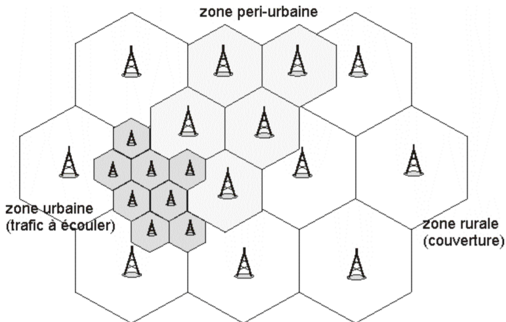
Figure II.10. Différents types de cellules selon la zone desservie
