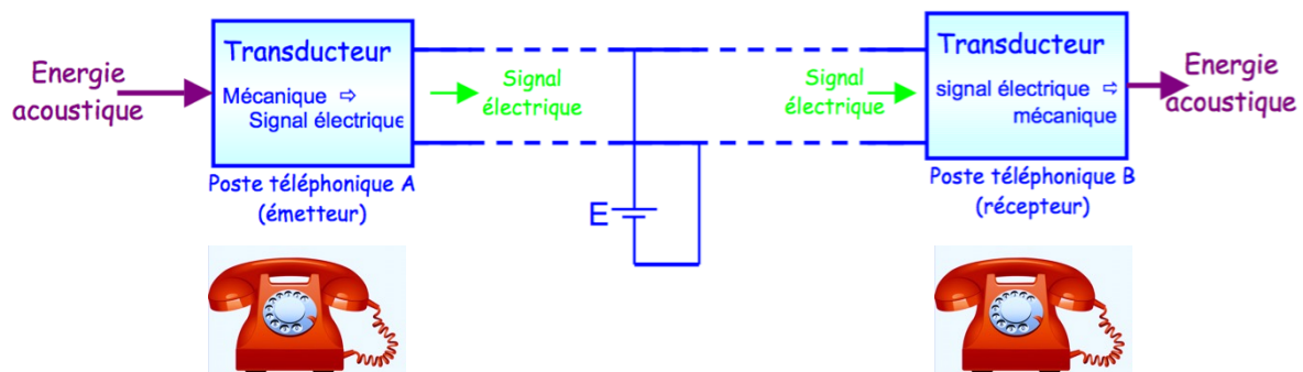
Figure II.1. Schéma de principe d'une liaison téléphonique élémentaire
