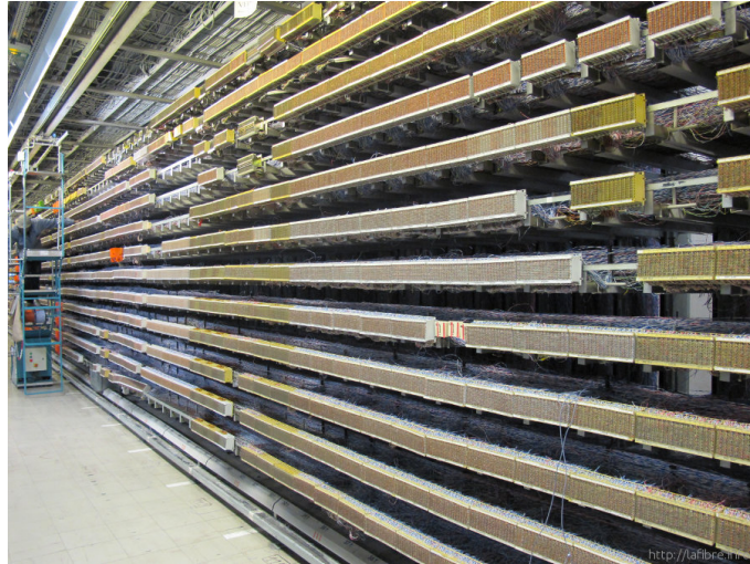
Figure II.6. Répartiteurs généraux
