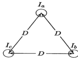
Fig.8. Ligne triphasée avec espacement équilibré.
