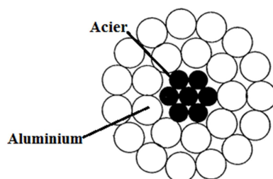
Fig.2 .Coupe transversale d'un conducteur renforcé d'acier, 7 brins d'acier, et 24 brins en aluminium.
