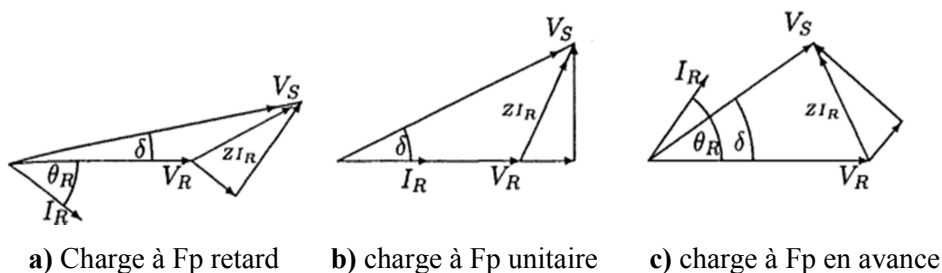
Fig. 19. Diagramme de phase pour une ligne courte.
