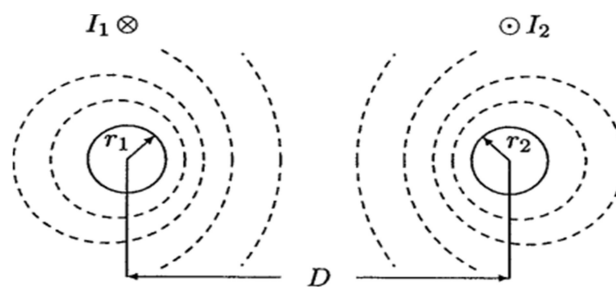
Fig.7. Ligne monophasé à deux fils.
