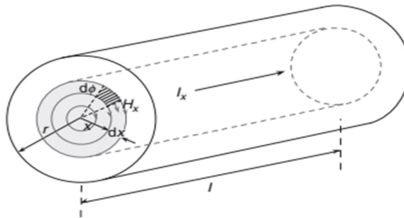
Fig.5. Flux magnétique interne.
