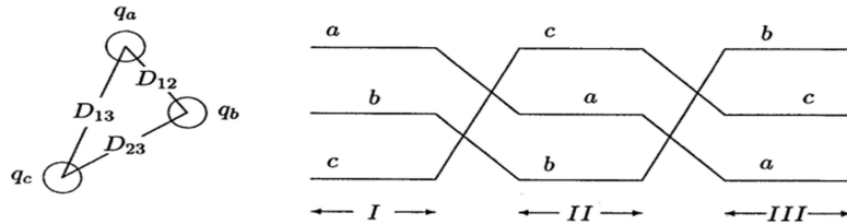
Fig.15. ligne de transport triphasée.
