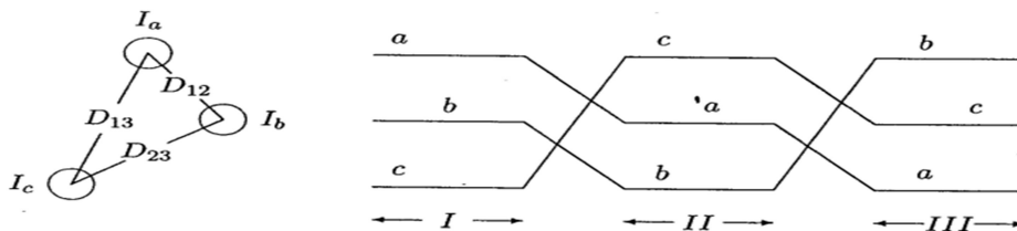
Fig.9. Ligne triphasée transposée.
