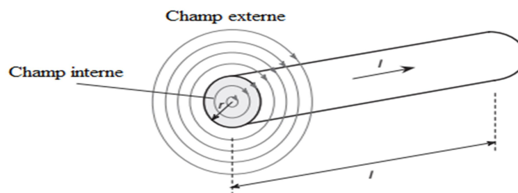
Fig.4. Lignes de flux magnétique concentriques externes et internes autour du conducteur.
