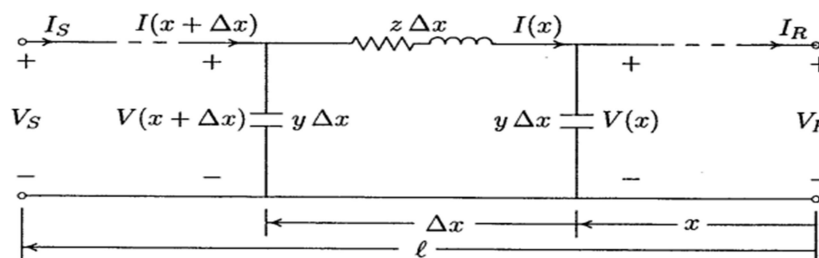
Fig.21. Ligne longue à paramètres distribués.
