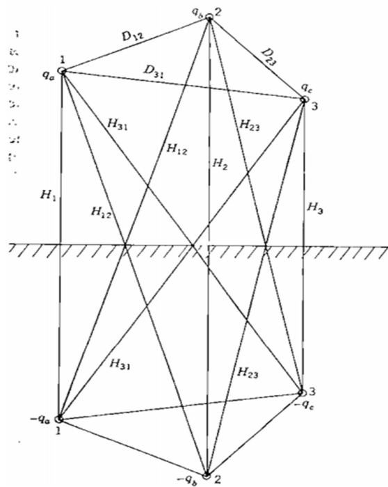
Fig.16. Ligne triphasée et son image.
