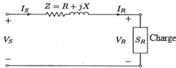
Fig.17. Modèle d'une ligne courte.
