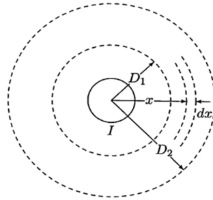
Fig.6. Liaison de flux entre D1 et D2.
