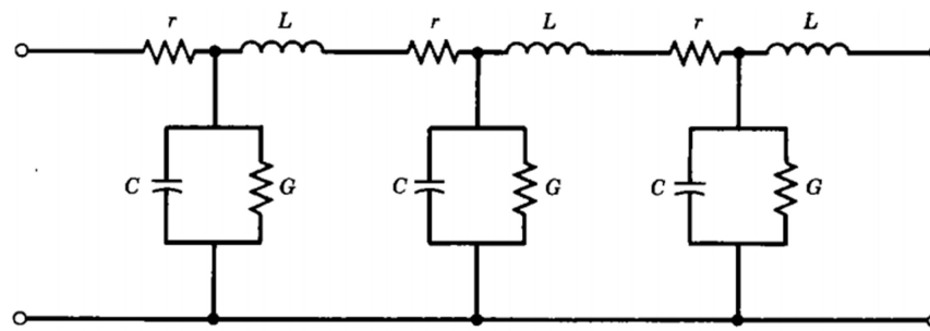
Fig.3. Circuit équivalent d'un circuit équivalent à constantes distribuées d'une ligne.
