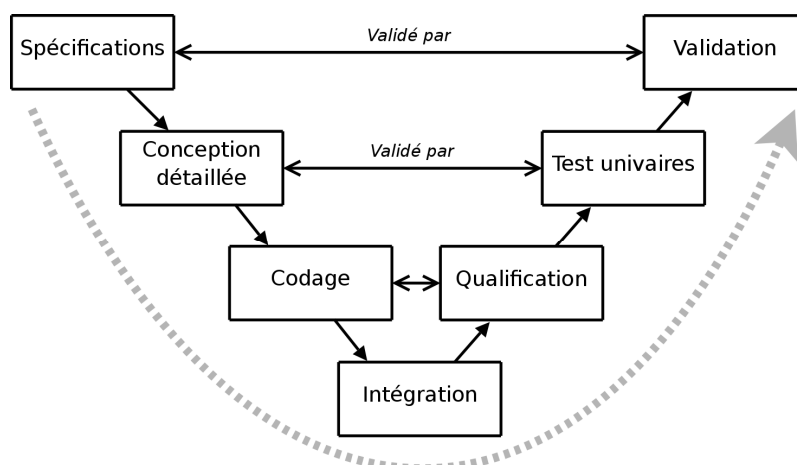
Figure 2: Modèle du cycle de vie en V
