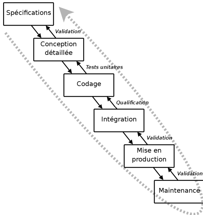
Figure 1 : Modèle du cycle de vie en cascade
